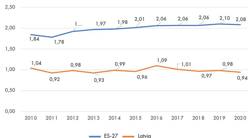
RESURSU PRODUKTIVITĀTE (EUR UZ KILOGRAMU)
