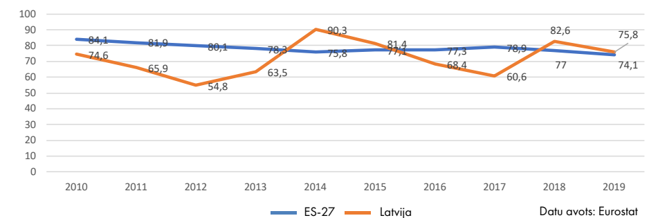
SILTUMNĪCAS EFEKTA GĀZU EMISIJAS GADĀ, IESKAITOT ZIZIMM SEKTORU (PRET EMISIJU APJOMU BĀZES GADĀ, 1990=100)
